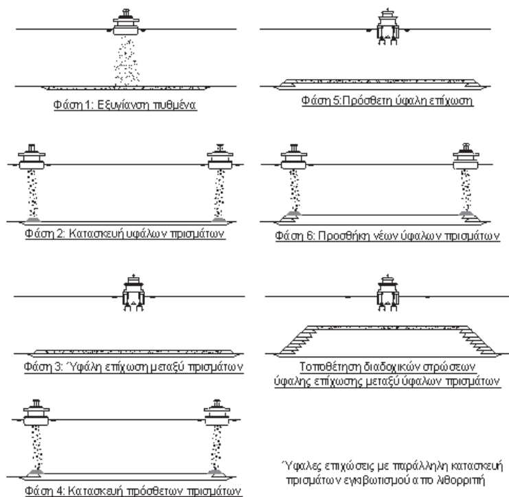
Σχήμα 1 – Κατασκευή υφάλων επιχώσεων με παράλληλη κατασκευή πρισμάτων εγκιβωτισμού από λιθορριπή
