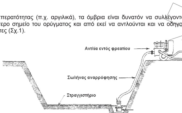
Σχήμα 1 - Άντληση στο χαμηλότερο σημείο του ορύγματος
