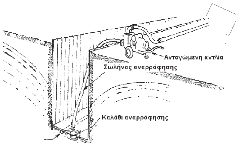
Σχήμα 3 - Αντληση από ορύγματα των οποίων οι παρειές αντιστηρίζονται με πασσαλοσανίδες ή μεταλλικά πετάσματα
