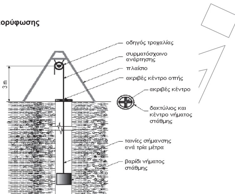
Σχήμα 2 - Διάταξη ελέγχου κατακορύφωσης υδρογεώτρησης
