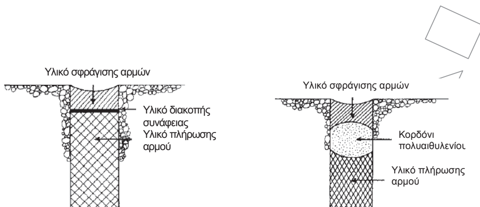
Σχήμα 1 – Τυπικές διατάξεις αρμών
