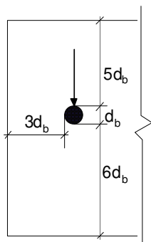
Σχ. Σ6.6: Ορισμός επικαλύψεων βλήτρου
