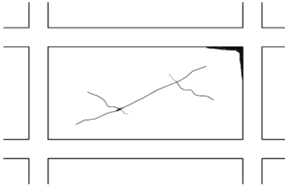
Σ2.2 : Σοβαρή βλάβη τοιχοπλήρωσης, ρωγμές > 5mm
