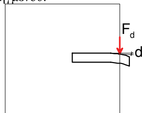
Σχ. Σ6.7: Παραμόρφωση βλήτρου
