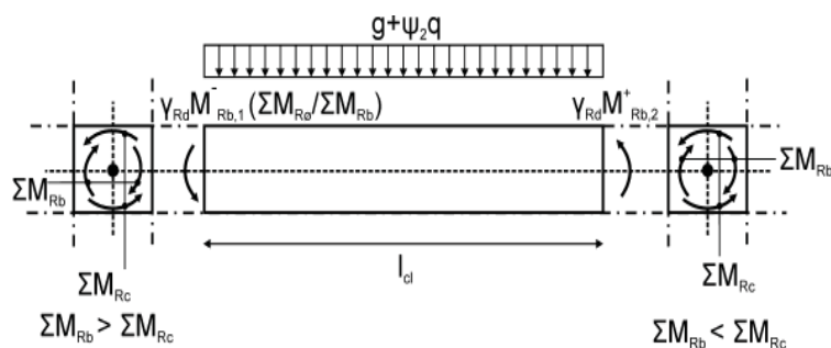
Σχ. Σ.9.2 Ενδεικτικό παράδειγμα καμπτικών αντιστάσεων στα άκρα δοκών για ικανοτικόν υπολογισμόν τέμνουσας δύναμης
