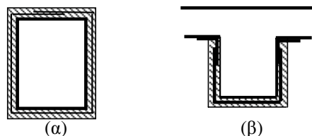
Σχ. Σ8.3: Ενδεικτικοί τρόποι ενίσχυσης σε διάτμηση έναντι ανεπάρκειας σε λοξή θλίψη: (α), Κλειστές ενισχύσεις, (β) Ανοικτές ενισχύσεις με ισχυρή σύνδεση στα άκρα
