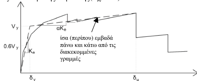
Σχ. Σ5.2 Εξιδανίκευση μιας (σχηματικής) καμπύλης αντίστασης της κατασκευής με διγραμμική καμπύλη
