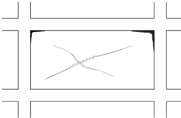
Σ2.3 : Βαριά βλάβη τοιχοπλήρωσης, ρωγμές > 10mm
