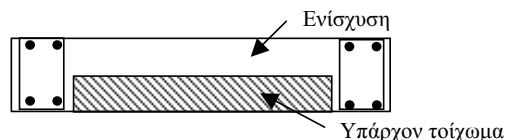
Σχ. Σ8.4: Ενδεικτική διάταξη μονόπλευρης ενίσχυσης τοιχώματος
