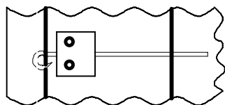
Σχ. Σ8.10: Ενδεικτική απεικόνιση αγκύρωσης οριζόντιων οπλισμών
