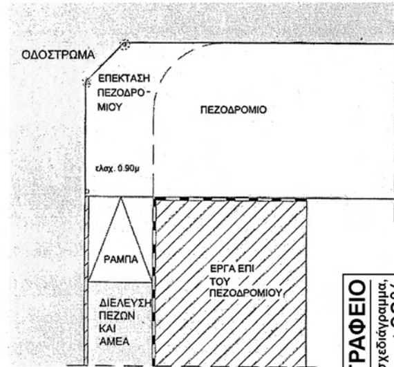
1η ΠΕΡΙΠΤΩΣΗ: Με σκαφη (ράμπα) ή υποβίβαση της γωνίας
