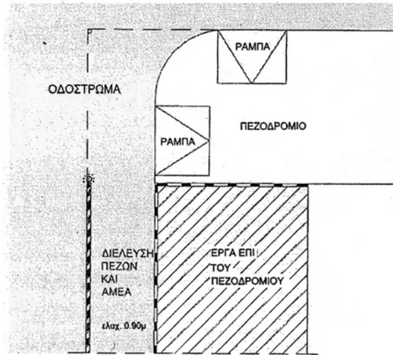
1η ΠΕΡΙΠΤΩΣΗ: Με σκαφη (ράμπα) ή υποβίβαση της γωνίας
